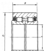
NNU4920WB-2LSV 型
