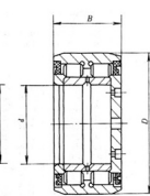
NNU4920WB-2LSV 型
