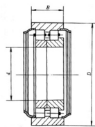
NNU4920-2Z 型 (172000 型)
