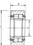
NNU4938-2Z 型 (462000 型)
