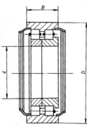
NNU4938-2Z 型 (172000 型)
