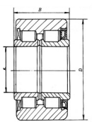
NNU4938-2LSV 型 (172000 型)
