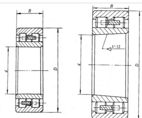
NNU4938 型 (482000 型)
