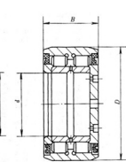
NNU4992WB-2LSV 型
