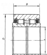
NNU4992WB-2LSV 型
