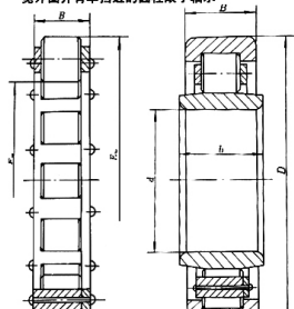
R200×00×00 型 (602000 型)
