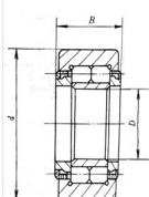
NNU4970-2Z 型 (462000 型)
