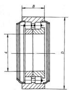
NNU4970-2Z 型 (172000 型)
