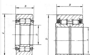
NNLT0000-2Z 型 (462000 型)
