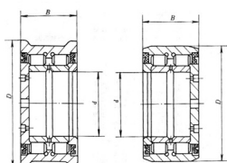
NNPT0000-2LSV 型
