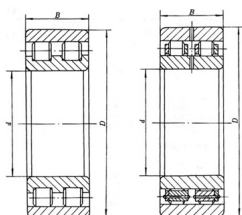
N40000V 型 (682000 型)
