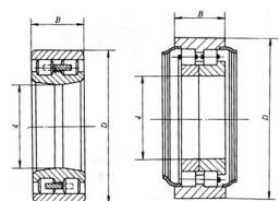
NNU4028X2-2K 型 (82000 型)
