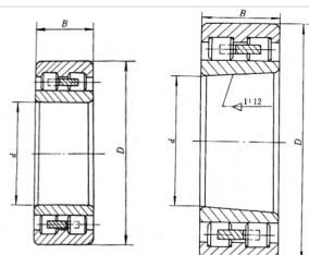
NNU4028X2 型 (482000 型)
