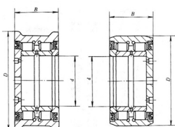
NNU4028X2-2LSV 型
