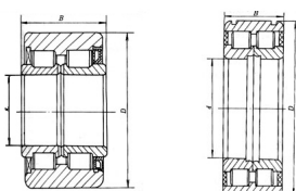
NNU4028X2-2LSV 型 (172000 型)
