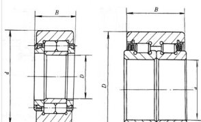
NNU4028X2-2Z 型 (462000 型)
