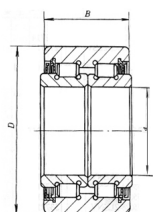
NN0000WB-2LSV 型
