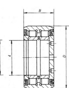
NNU4156WB-2LSV 型
