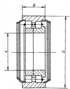
NNU4156-2Z 型 (172000 型)
