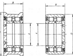
NN4960V-2LSV 型
