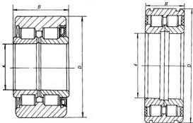
NN4960V-2LSV 型 (1272000 型)
