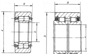
NN4960V-2Z 型 (462000 型)
