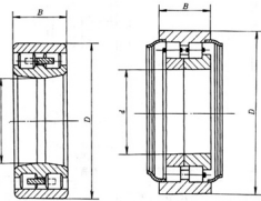
NN4960V-2K 型 (82000 型)
