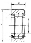
NN49000-2Z型 (462000型)
