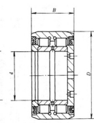
NNFP0000-2LSV 型
