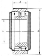
NN0000-2Z 型 (172000 型)
