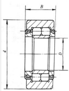
NNLP0000-2Z 型 (462000 型)
