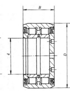
NNFP0000-2LSV 型
