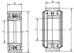
NN0000-2K 型 (82000 型)
