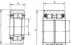
NNUPN33/114.3-2LSV 型 (462000 型)
