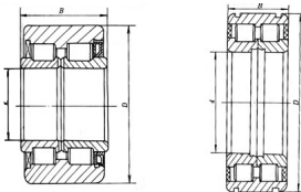
NN0000-2LSV 型 (172000 型)
