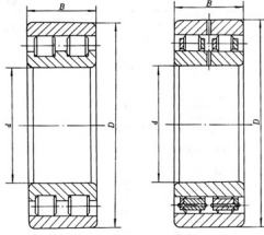
NN40000V (682000 型)
