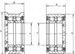
NNFP0000-2LSV 型
