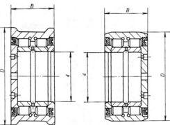
NNJ0000-2LSV 型
