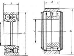
NNJ0000-2K 型 (82000 型)
