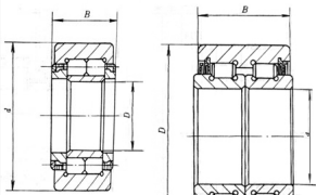
NNJ0000-2Z 型 (462000 型)
