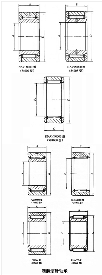
满装滚针轴承
